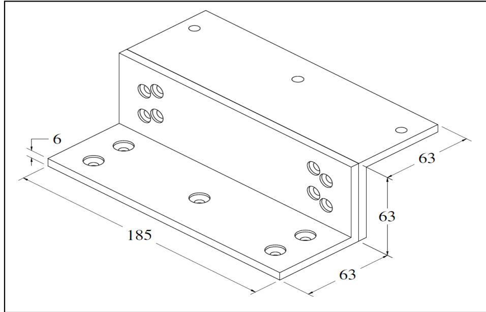
1200 LBS WATER PROOF EM LOCK Z-545 BRACKET
